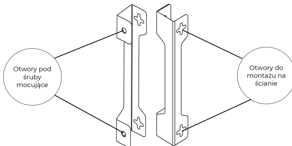
2 – Wsporniki do montażu na ścianie
