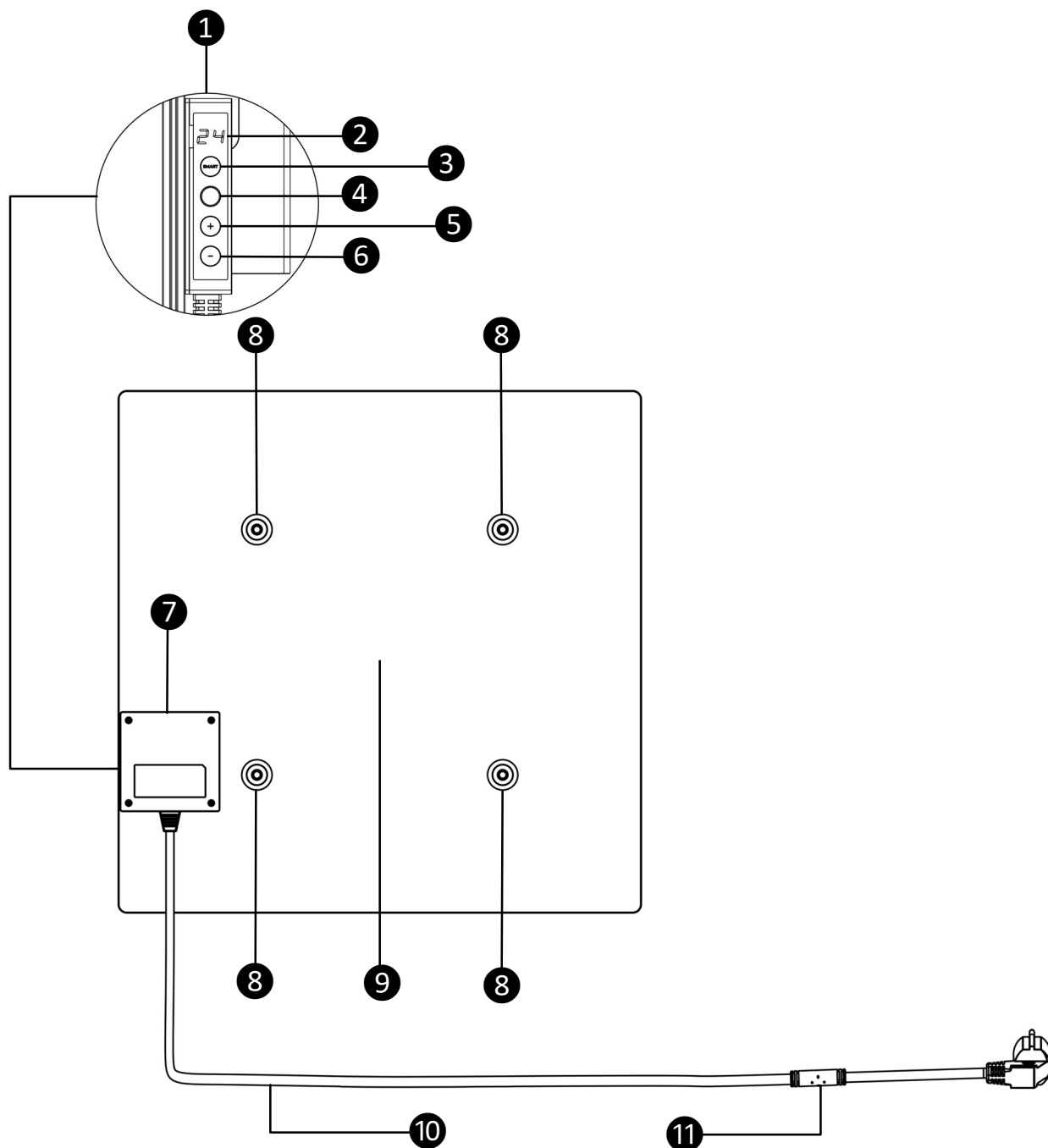
Rysunek 6 – Elementy urządzenia (AGH0011S–AGH0013S)
