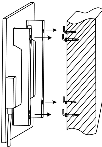
Rysunek 23 – Montaż na hakach (AGH0011S–AGH0013S)
