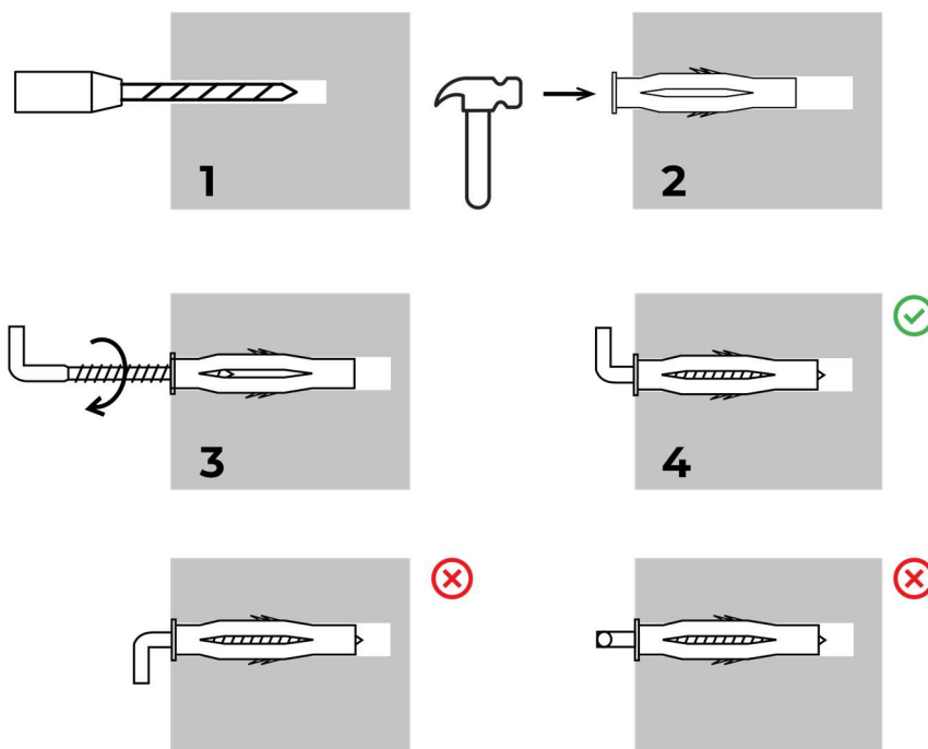
Rysunek 22 – Montaż kołków rozporowych i haków
