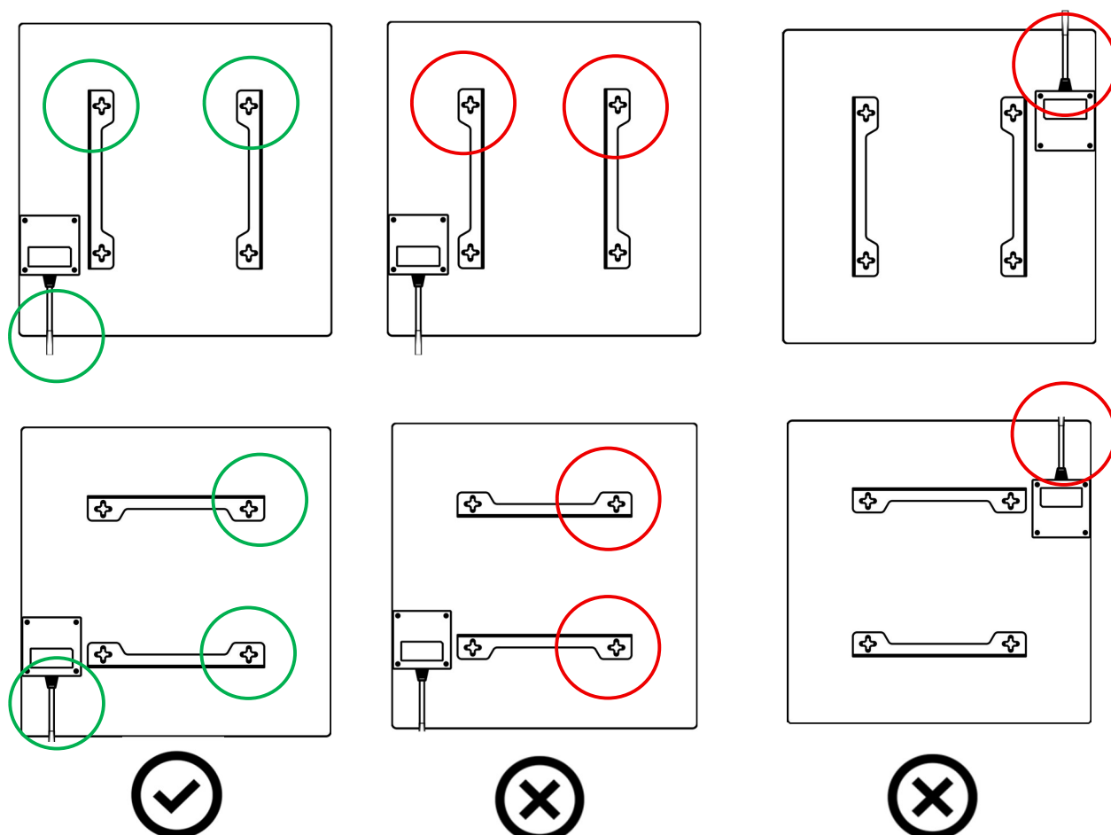
Rysunek 19 – Orientacja wsporników (AGH0011S–AGH0013S)
