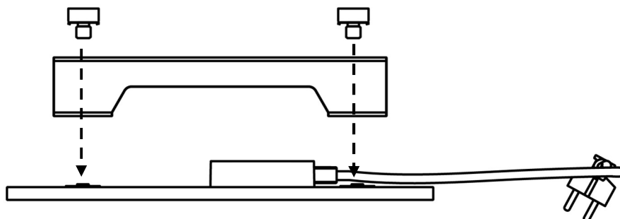
Rysunek 14 – Mocowanie wsporników (AGH0001S, AGH0002S, AGH0003S–AGH0006S)
