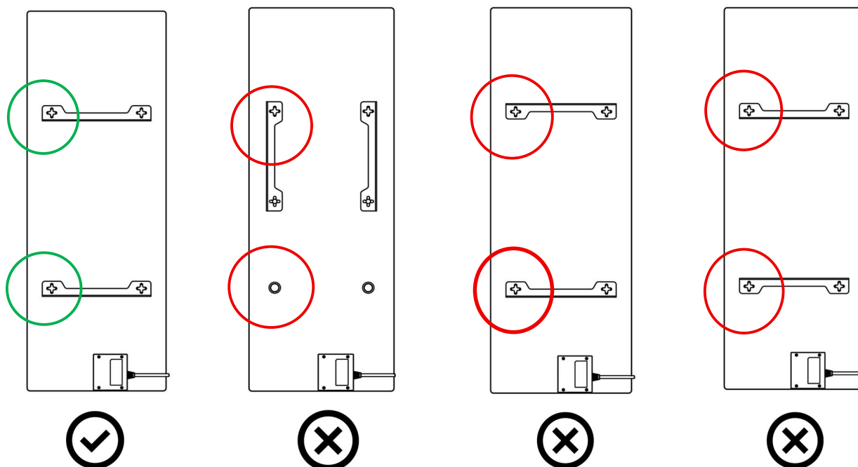
Rysunek 13 – Pionowa orientacja grzejnika (AGH0001S, AGH0002S, AGH0003S–AGH0006S)
